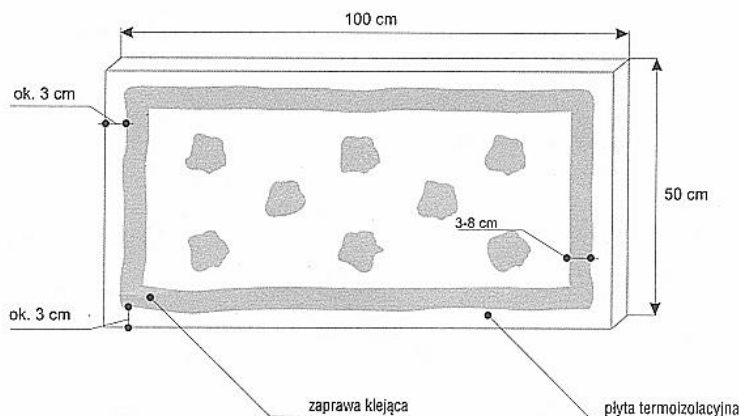
Fig.1 - Przykładowy sposób rozmieszczenia zaprawy klejącej na płycie styropianowej
