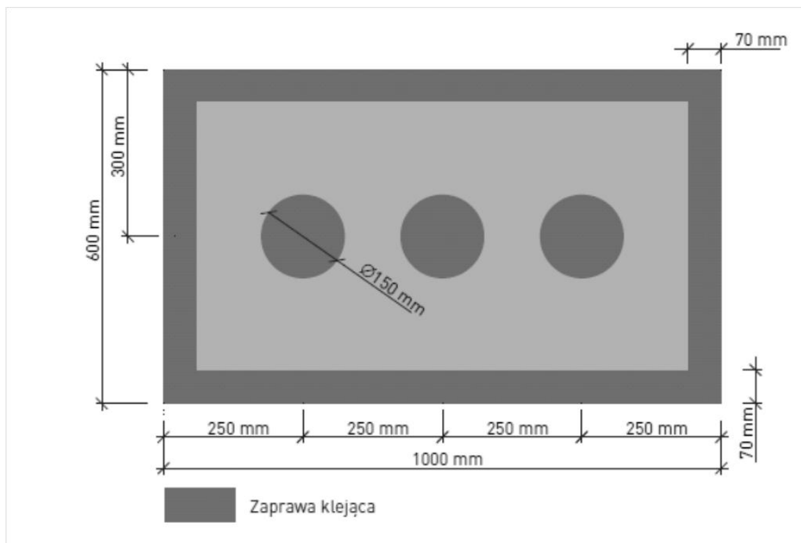
Fig. 1 Zasady nakładania kleju w metodzie obwodowo-punktowej na płycie).
