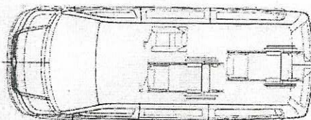
WJAZD TYŁEM PRZEZ DRZWI SKRZYDŁOWE - 2 wózki
